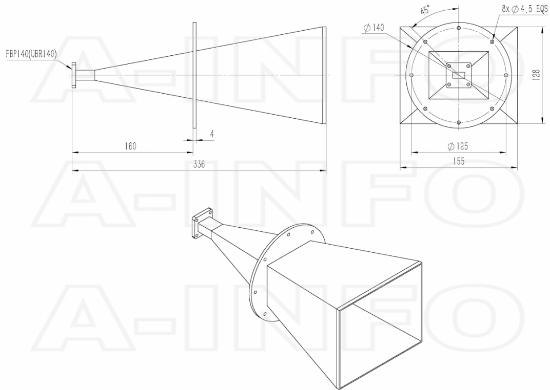
FBP140 Output (P/N: LB-62-25-A2)
